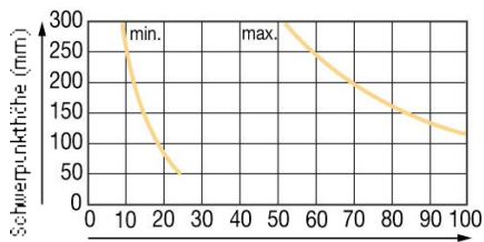
Kameraplattform Counterbalance
