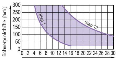
Kameraplattform Counterbalance
