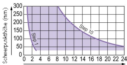
Kameraplattform Counterbalance
