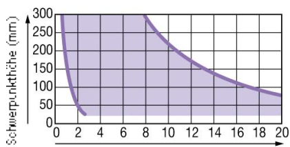
Kameraplattform Counterbalance
