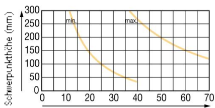
Kameraplattform Counterbalance
